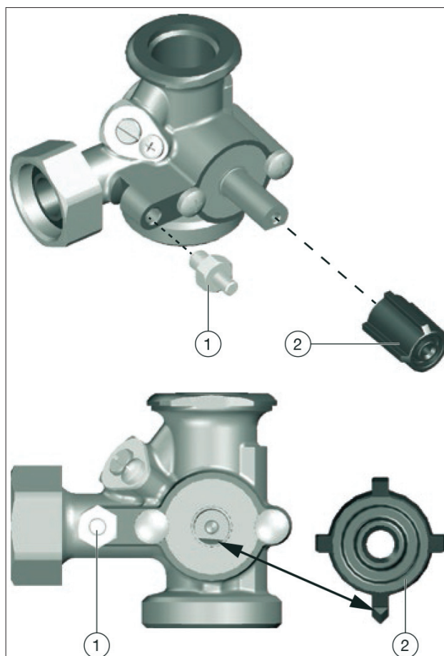
Рис. 3: Установка
