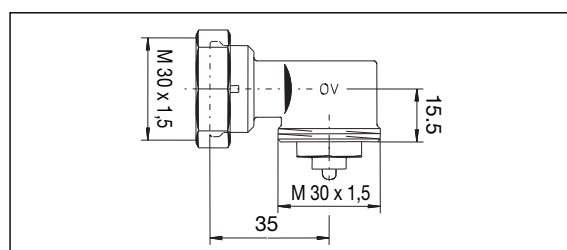
Haakse adapter art.nr. 101 14 50
