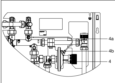
Abb. 8.2 Entlüftung
