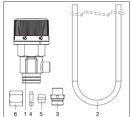
Abb. 6.1 Lieferumfang
