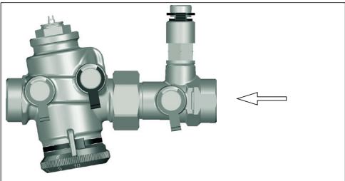
Abb. 13: Überwurfmutter anziehen
