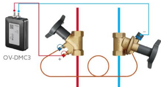
Bild 9: Kopplingsschema OV-DMC 3
