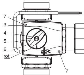
Schalter S1 in Drehrichtung
