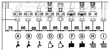
Fig. 4.3 Misura collegamenti
