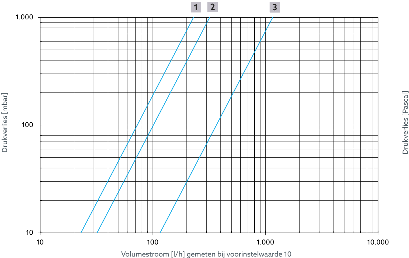
Afb. 18: Volumestroom Thermische regeling voor artikelnummers 4202553 en 4202753
