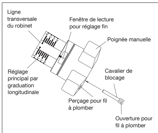
Poignée manuelle
