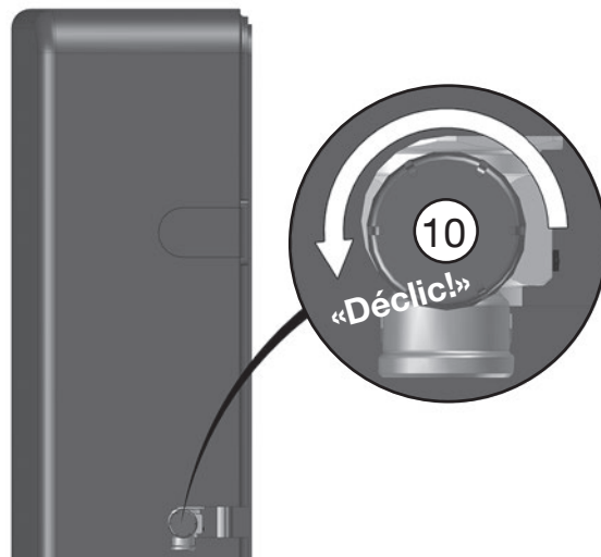
Fig. 6.4: Tourner la soupape de sécurité dans le sens inverse des aiguilles d'une montre
