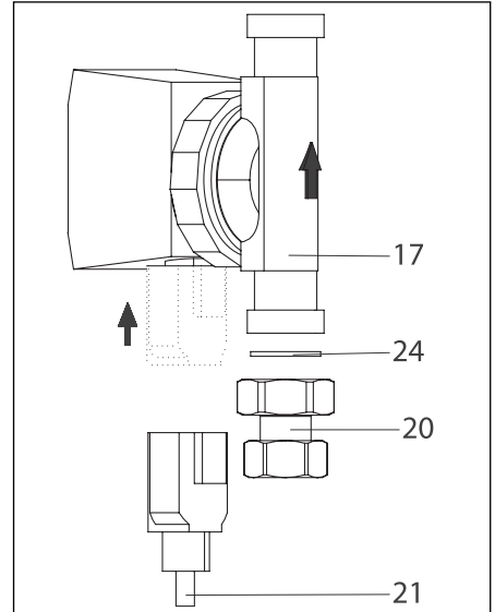
Abb. 6.2 Pumpenausrichtung
