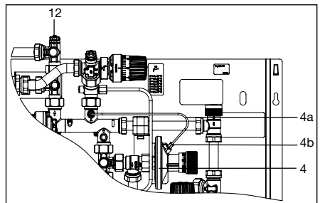
Abb. 8.2 Entlüftung
