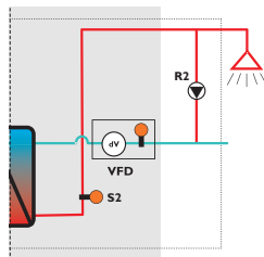
circuit secondaire
