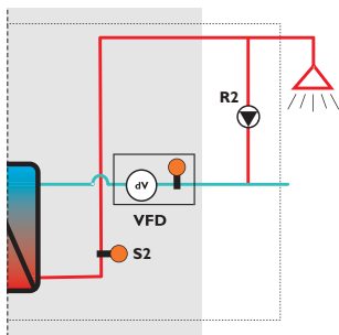
circuit secondaire
