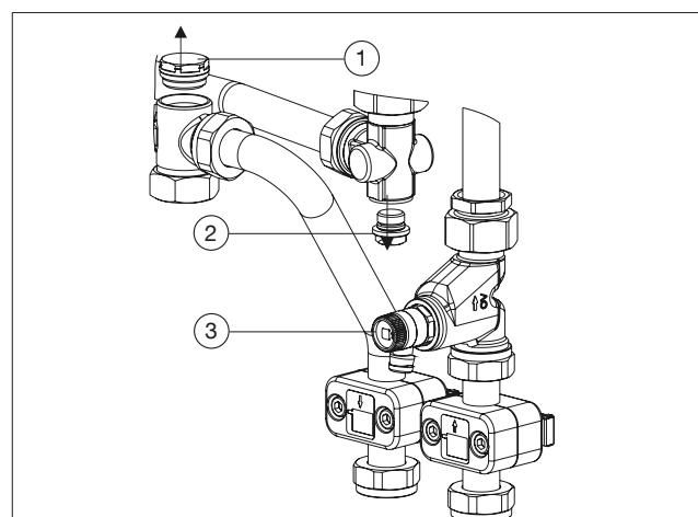
Fig. 6: Démontage des bouchons Regudis W-HTO
