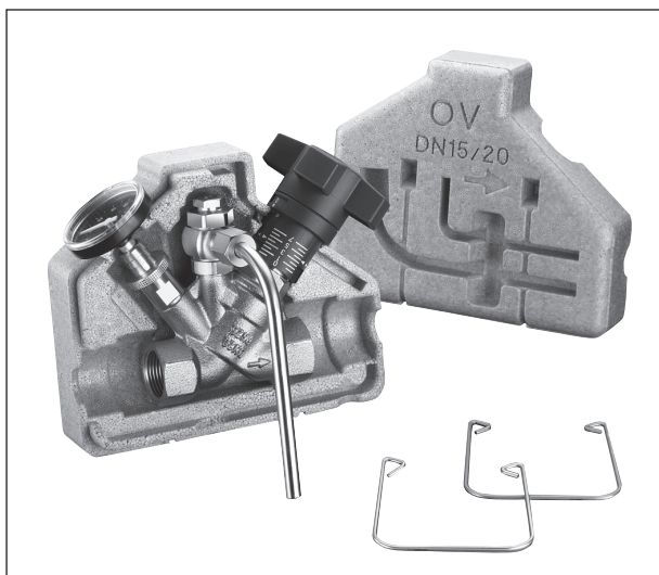
„Aquastrum C“ mit Isolierung und „Aquastrum P“
