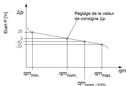
Écart P le plus faible pour un réglage moyen de la valeur de consigne ( q_{m\text{nom}} )
