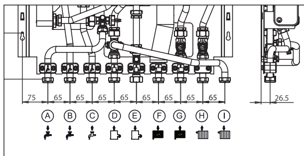
Anschlussmaße
