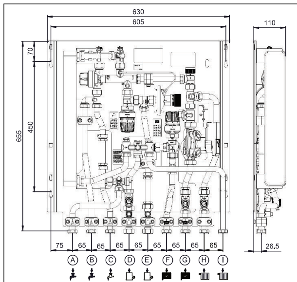
Abmessungen mit gemischtem Heizkreis und Hochtemperaturkreis
