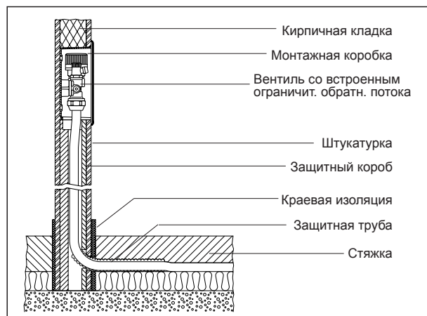
„Unibox E RTL“, глубина 57 мм
