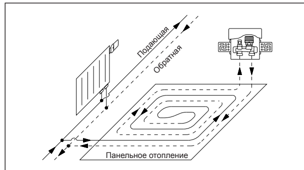
Схема монтажа для регулирования температуры панельного отопления посредством ограничения температуры обратного потока
