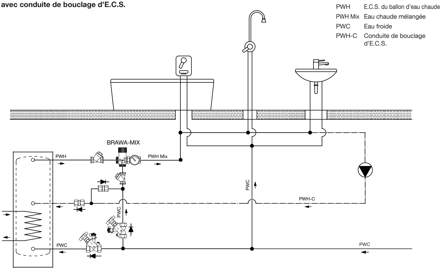
Exemple d’application de la vanne «Brawa-Mix» dans une installation d’eau potable avec conduite de bouclage d’E.C.S.
