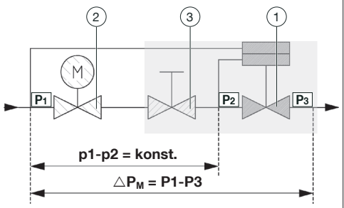
Abb. 3: Schéma fonctionnel du « Cocon QTZ »
