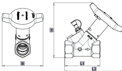
Abb. 2: Encombremens vue de côté / vue de face - Version avec filetage
