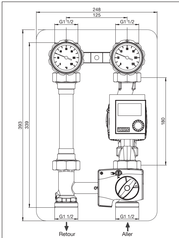
Encombrements Regumat 180 DN 25
