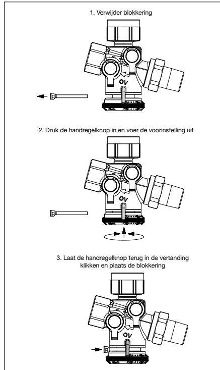
Afb. 7 Debietinstelling
