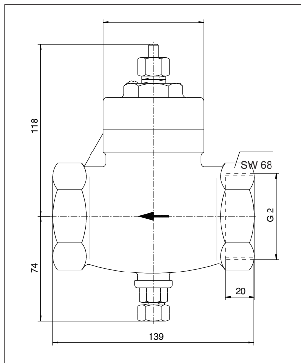
Dimensioni
