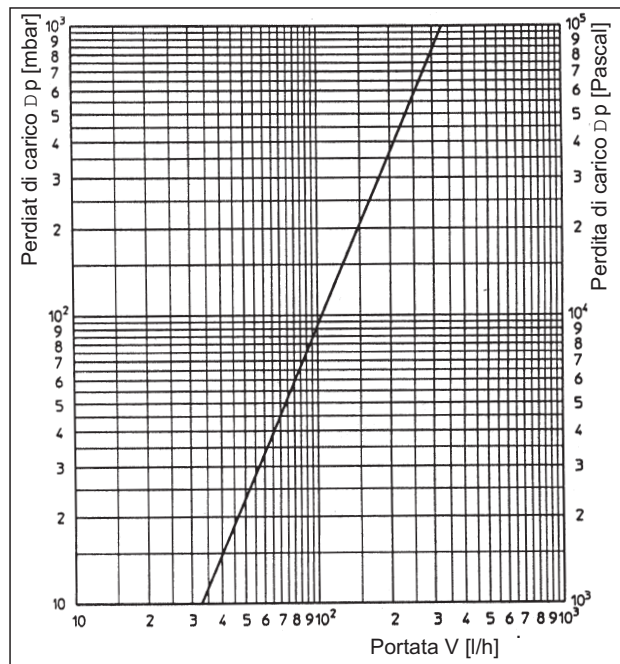
Portata minima a cono valvola chiuso (6)
