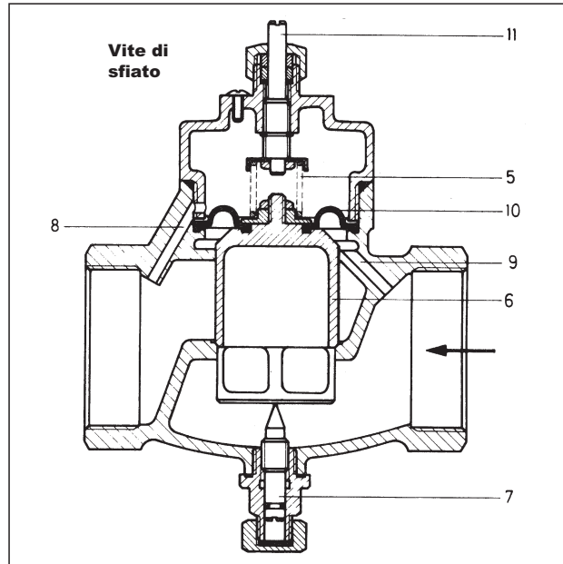
Sezione
