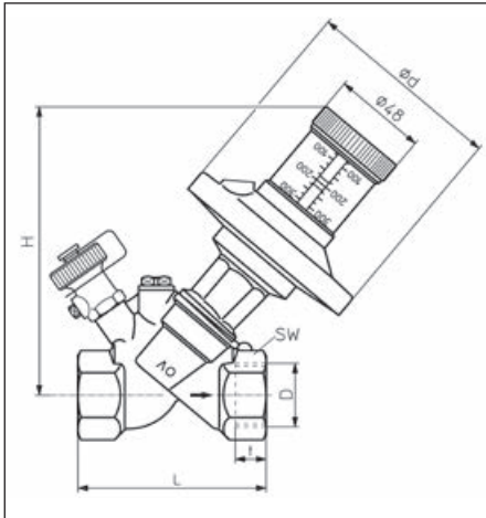
Fig. 4.1 Régulateur 1064904 – 16 filetage femelle NPT des deux côtés
