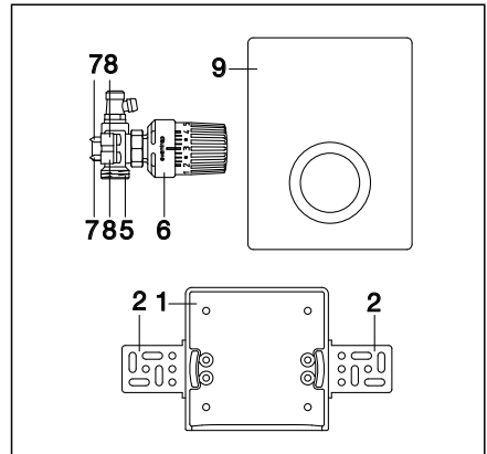
Komponenten Umrüstsatz
