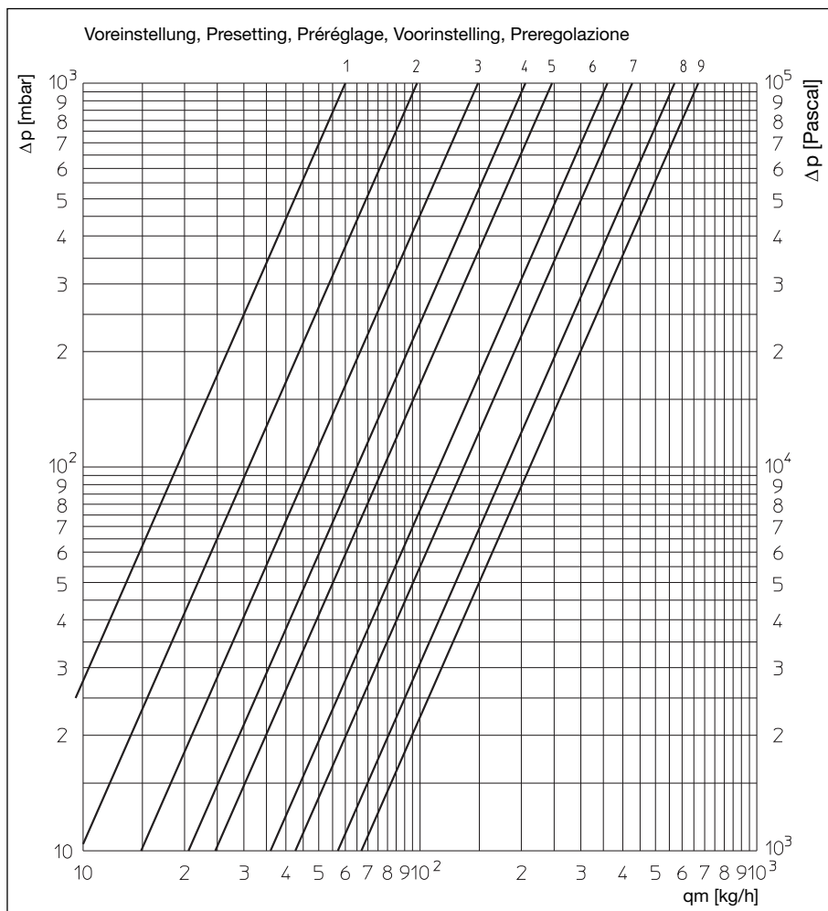
Druckverlustdiagramm „Unibox T“ mit Ventileinsatz der „Baureihe AV9“ bei 2 K P-Abweichung
