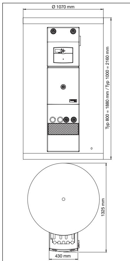
Fig. 2 Dimensioni
