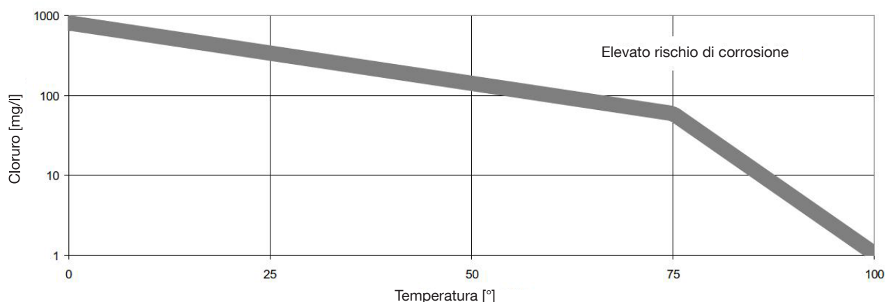
Contenuto di cloruro ammissibile a seconda della temperatura
