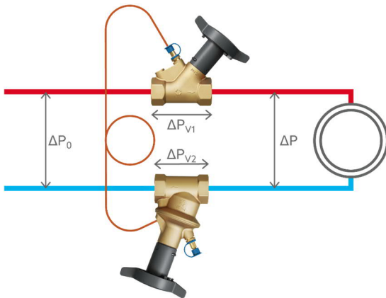
Schemat ideowy
