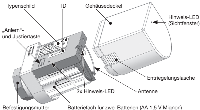
Abb. 4: Innenansicht der Funk-Stellantriebe „mote 320“:
