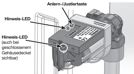
Abb. 18: Hinweis-LEDs am Funk-Stellantrieb „mote 320“ nach „Justierfahrt“
