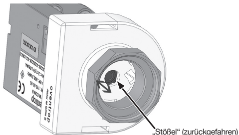
Abb. 11: Montageposition des Stößels des Funk-Stellantriebs „mote 320“
