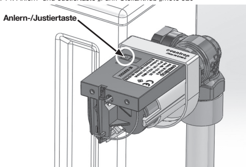
Abb. 14: Anlern- und Justiertaste „Funk-Stellantrieb „mote 320“
