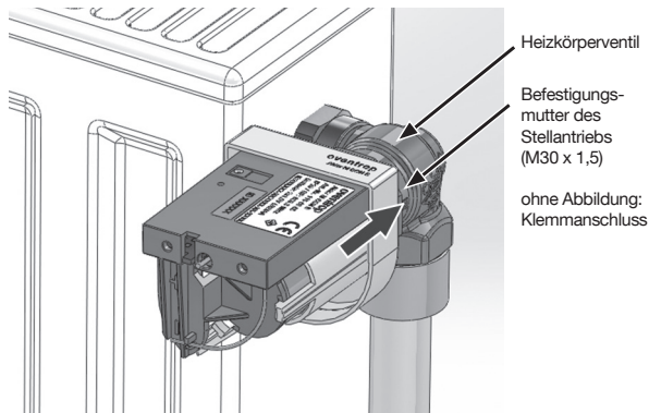
Abb. 10: Montage des Funk-Stellantriebs „mote 320“ an Heizkörperventil
