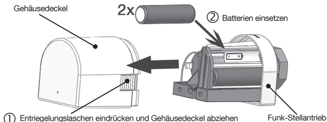
Abb. 9: Batterieeinsatz im „Funk-Stellantrieb „mote 320“
