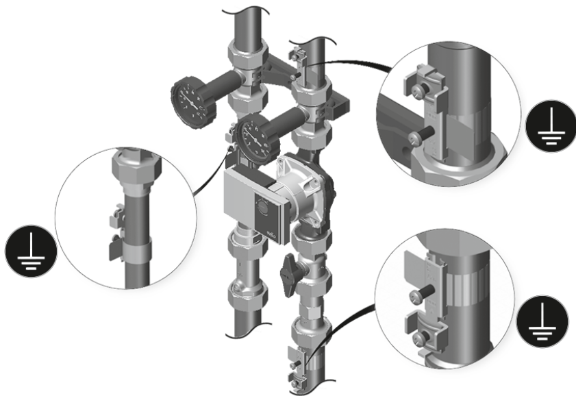
Рис. 26 Выравнивание потенциалов/заземление монтажа установки со стальной трубной обвязкой
