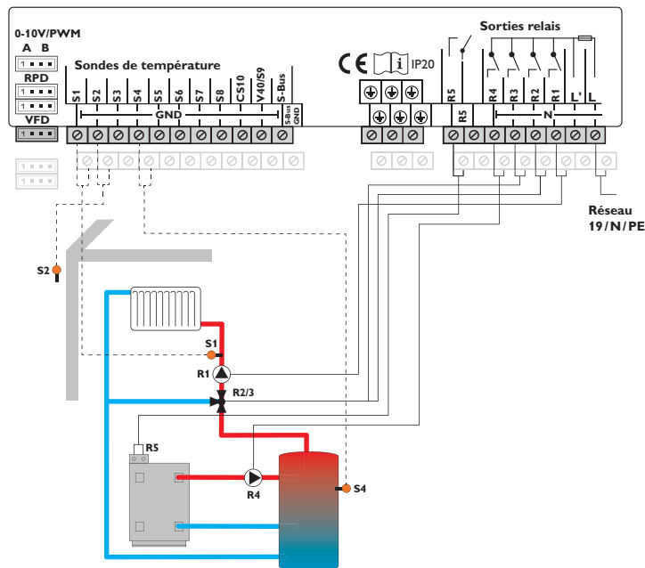
Schéma 3: circuit de chauffage mélangé avec chauffage d'appoint (demande ou pompe de charge de la chaudière)
