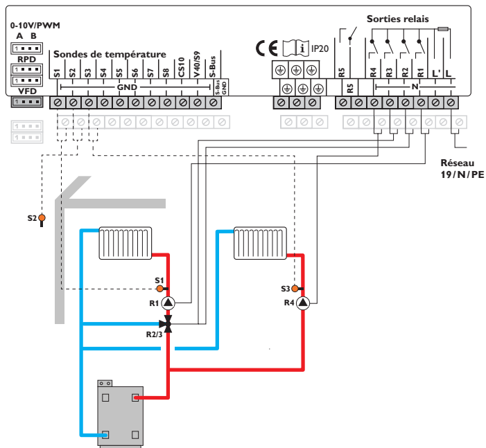
Schéma 6: circuit de chauffage mélangé et circuit de chauffage direct
