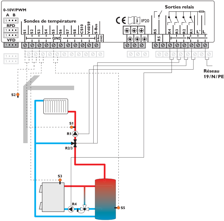
Schéma 8: circuit de chauffage mélangé avec chaudière à combustible solide
