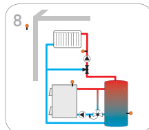
Circuit de chauffage mélangé avec chaudière à combustible solide
