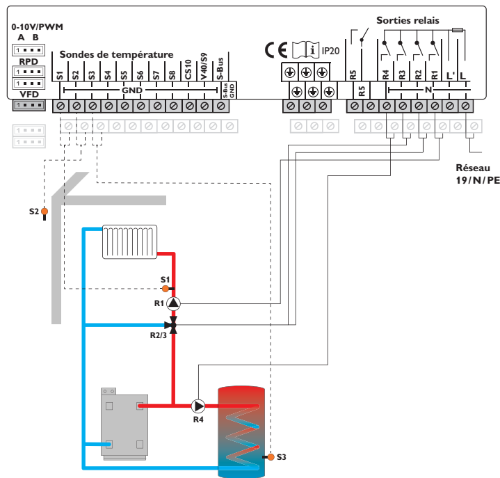
Schéma 4: circuit de chauffage mélangé avec chauffage de l'ECS
