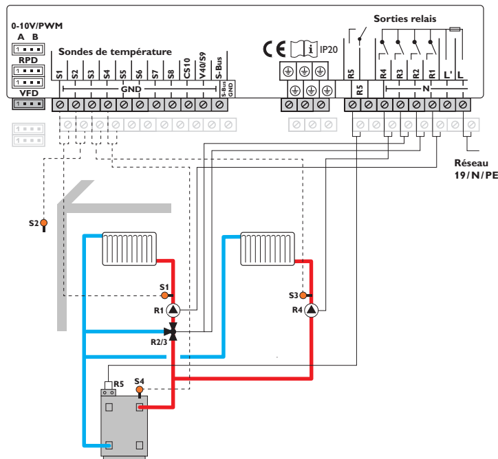
Schéma 7: circuit de chauffage mélangé et circuit de chauffage direct avec chauffage d'appoint (demande)
