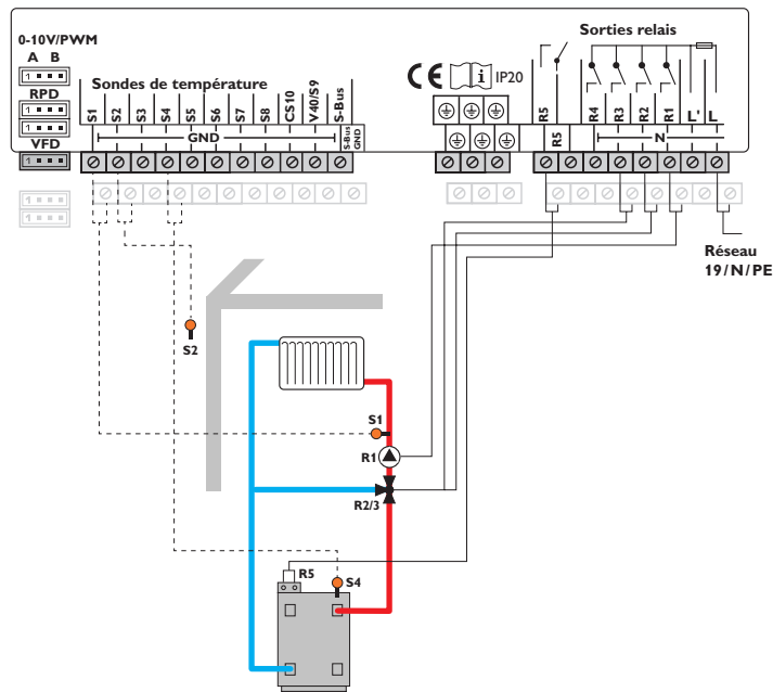
Schéma 2: circuit de chauffage mélangé avec chauffage d'appoint (demande)
