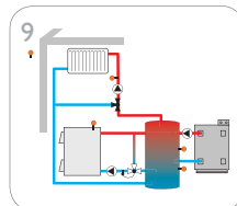
Circuit de chauffage mélangé avec chaudière à combustible solide et chauffage d'appoint
