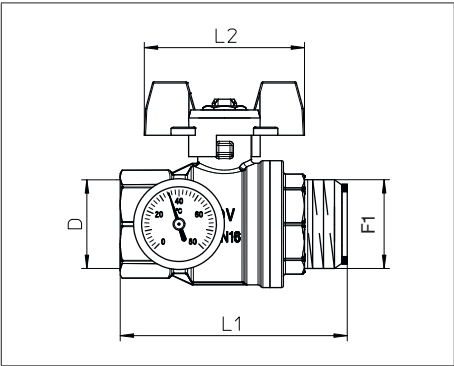
Fig. 8: Dimensiuni robinet sferic
