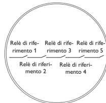
2. In serie (AND)
