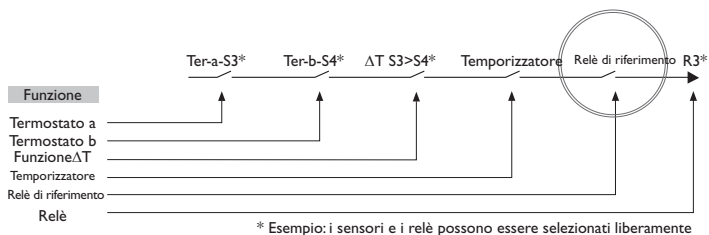
Relè di riferimento
