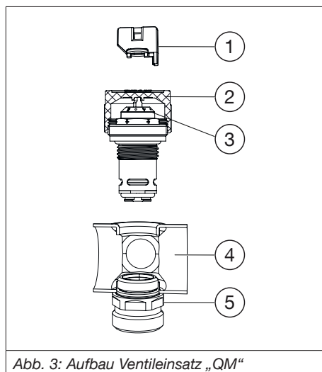
Abb. 3: Aufbau Ventileinsatz „QM“
