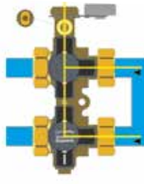
Izolarea și golirea consumatorului
