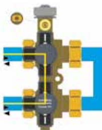
Funcționare în baipas
