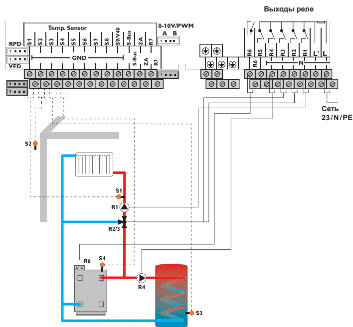
Схема 5: смешанный нагревательный контур с нагревом технической воды и дополнительным нагревом (запрос для нагревательного контура и технической воды)
