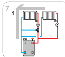
Смешанный и несмешанный нагревательный контур с дополнительным нагревом
