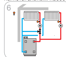
Смешанный и несмешанный нагревательный контур
