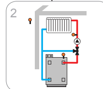
Смешанный нагревательный контур с дополнительным нагревом
