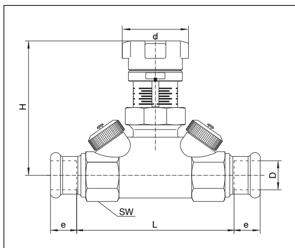
Maße „Hycococon VTZ“
