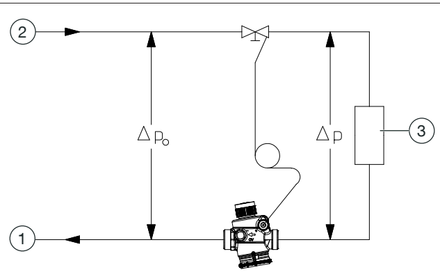
Fig. 4 : Exemple d'installation
