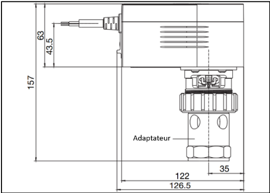
Encombrements du moteur réf. 1158011
