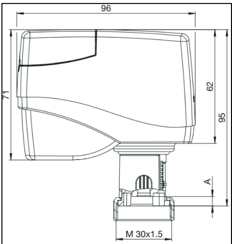
Encombrements du moteur réf. 1158012/13
