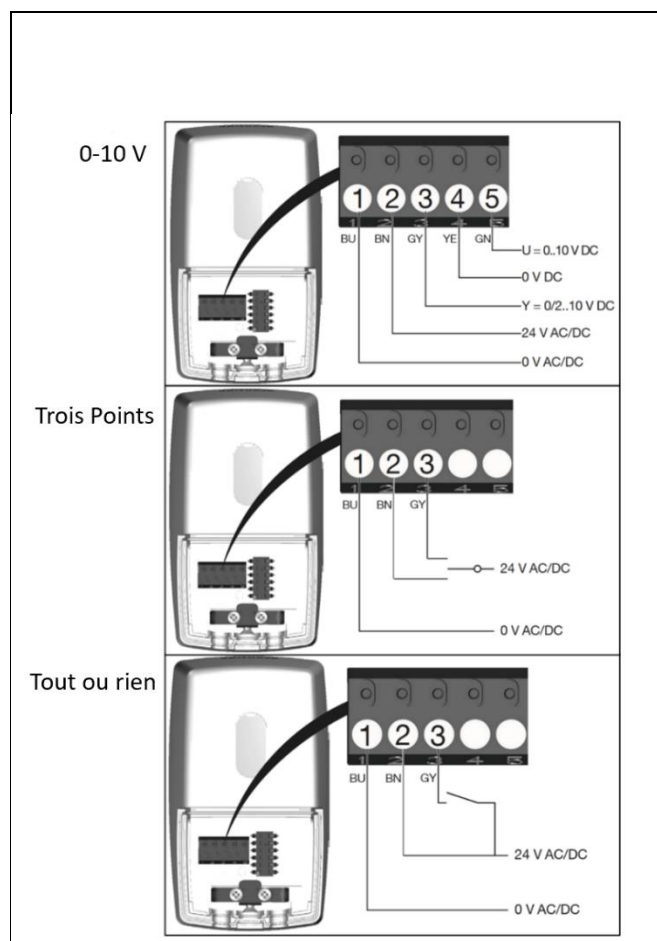
Schémas électriques réf. 1158012/13, trois points réf 1158012
