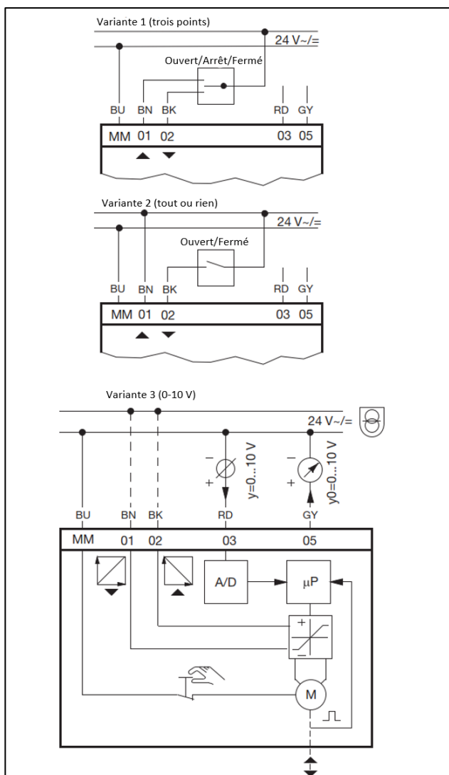
Schémas électriques réf. 1158011
