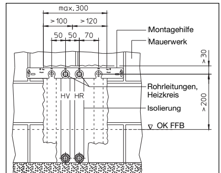
Abb. 7 Wandansicht, Heizkreisanschluss
