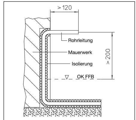
Abb. 6 Schnitt, Heizkreisanschluss
