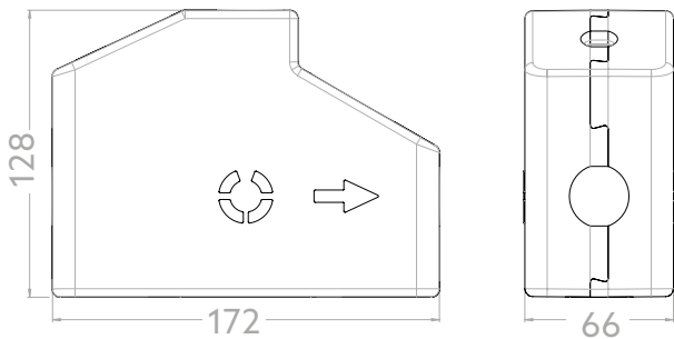
图 5： 绝缘壳
