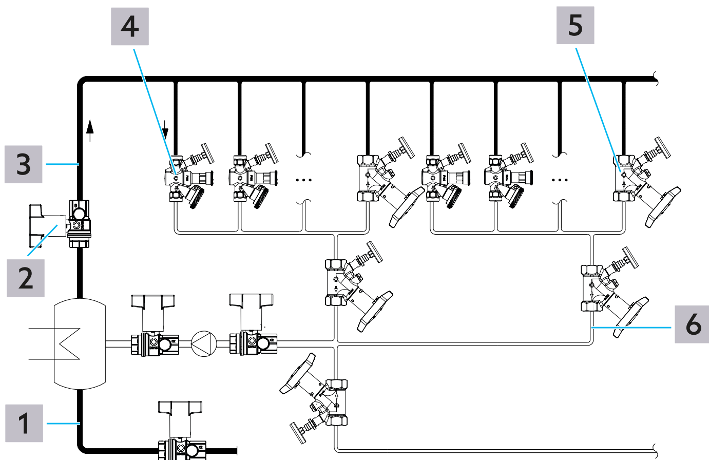
Рис. 4: Схема системы
