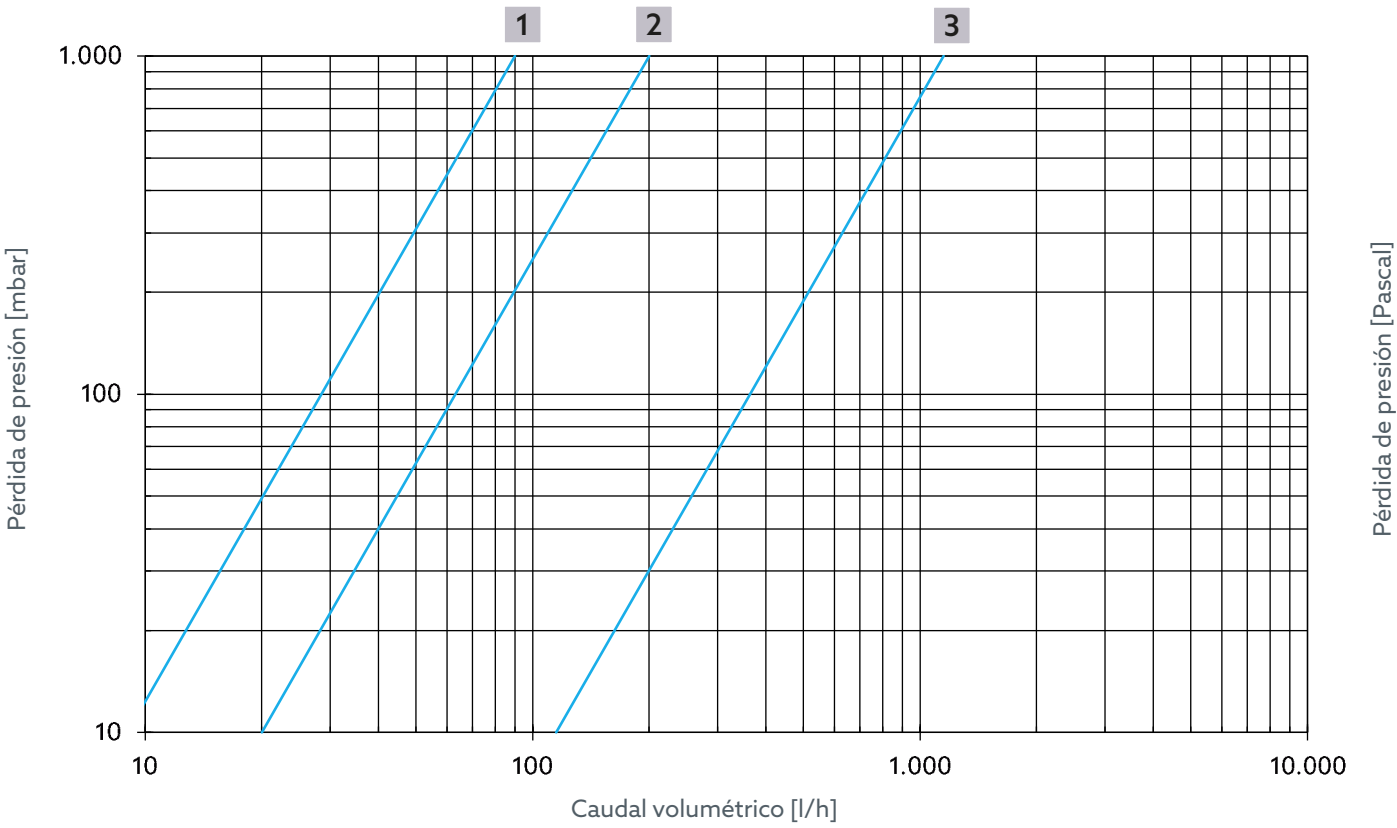
Fig. 9: Caudal volumétrico control térmico para los artículos n.º 4202904
