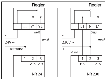
Abb. 5.3 Anschluss-Schema Dreipunktsteuerung
