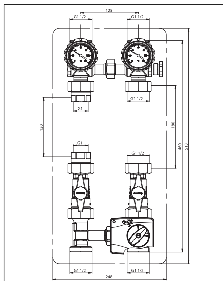
Fig. 4.2 Dimensioni per contacalorie 130 mm
