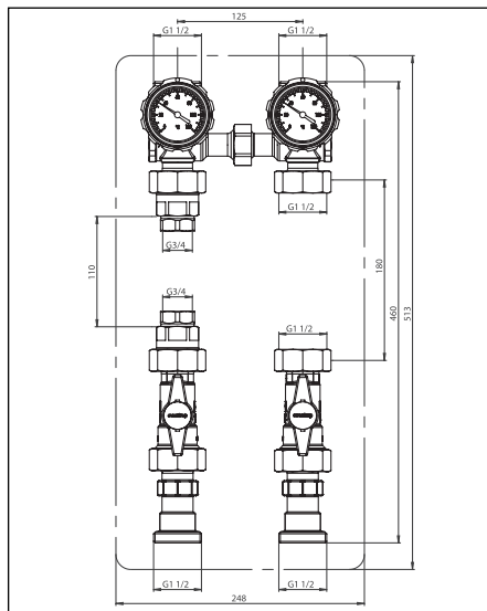
Fig. 4.1 Dimensioni per contacalorie 110 mm
