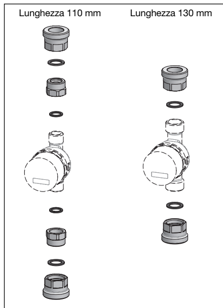
Fig. 5.5 Montaggio kit d'installazione contacalorie
