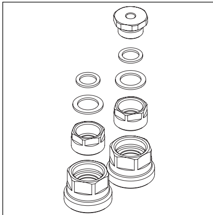
Abb. 5.4 Wärmemengenzähler-Einbauset
