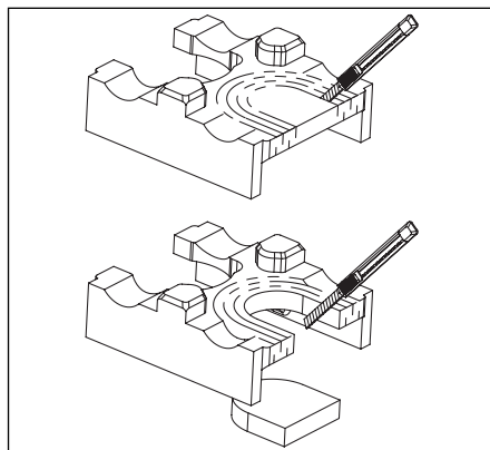
Fig. 5.6 Inserto con apertura per contacalorie
