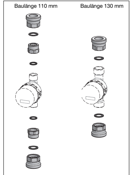
Abb. 5.5 Montage Wärmemengenzähler-Einbauset
