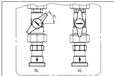
Abb. 5.1 Sperrventil geöffnet
