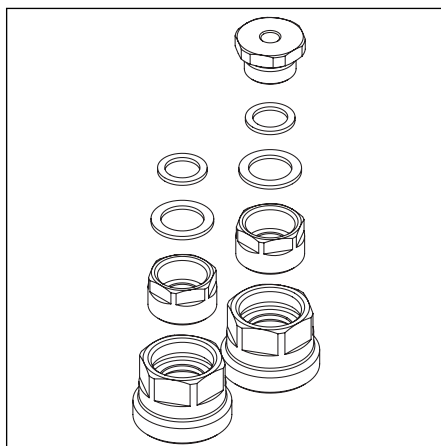
Fig. 5.4 Kit installazione del contacalorie
