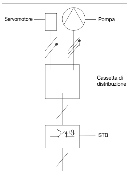
Fig. 4.1 Schema cablaggi
