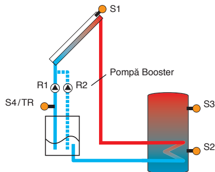
Exemplu de schemă pentru o instalație de purjare înapoi (R2 = pompă Booster)
