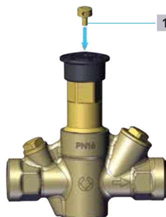
Ryc. 7: Zablokowanie wartości zadanej temperatury
