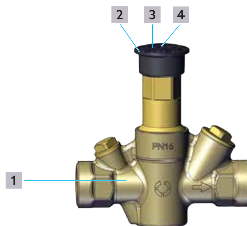
Obr. 1: Konštrukcia
