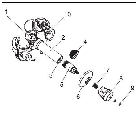
Рис. 6.1 Вентиль UP с защитной гильзой
