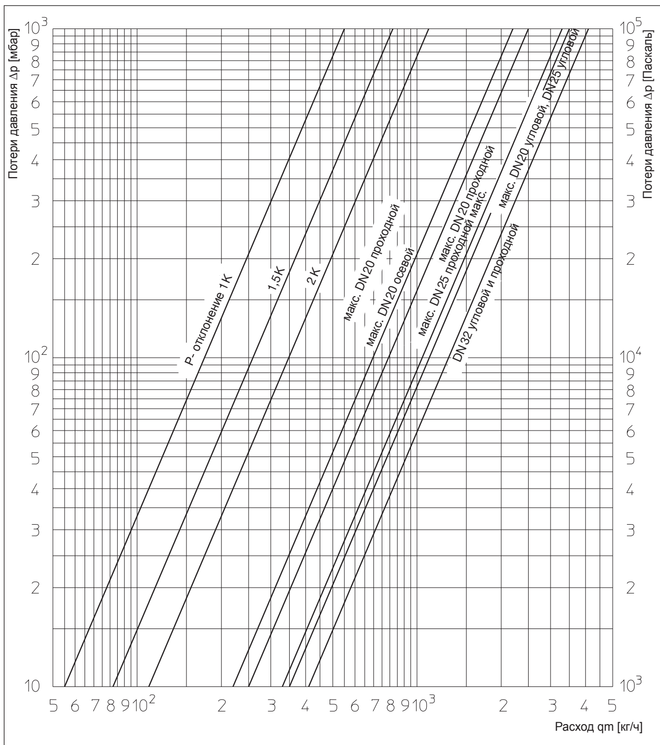
Диаграмма 2 Термостатические вентили Oventrop серии, „А“, DN 20-DN 32 и „RF“, DN 20 Все исполнения, Р-отклонение от 1 до 2 К и kvs.
