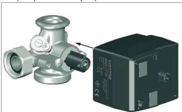
Рис. 4: Установить сервомотор
