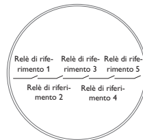
2. In serie (AND)
